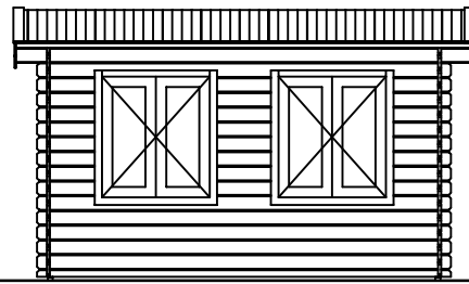
(L) Zijaanzicht / Side view / Seiten ansicht
