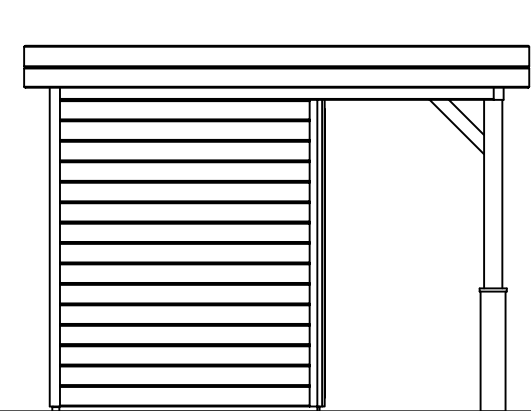
(L) Zijaanzicht / Side view / Seiten ansicht
